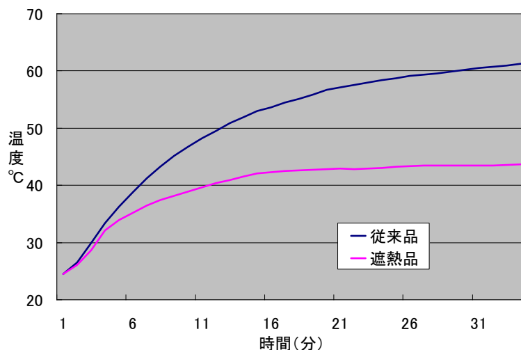
水性遮熱防水コートと従来の防水コートによる温度差の比較
